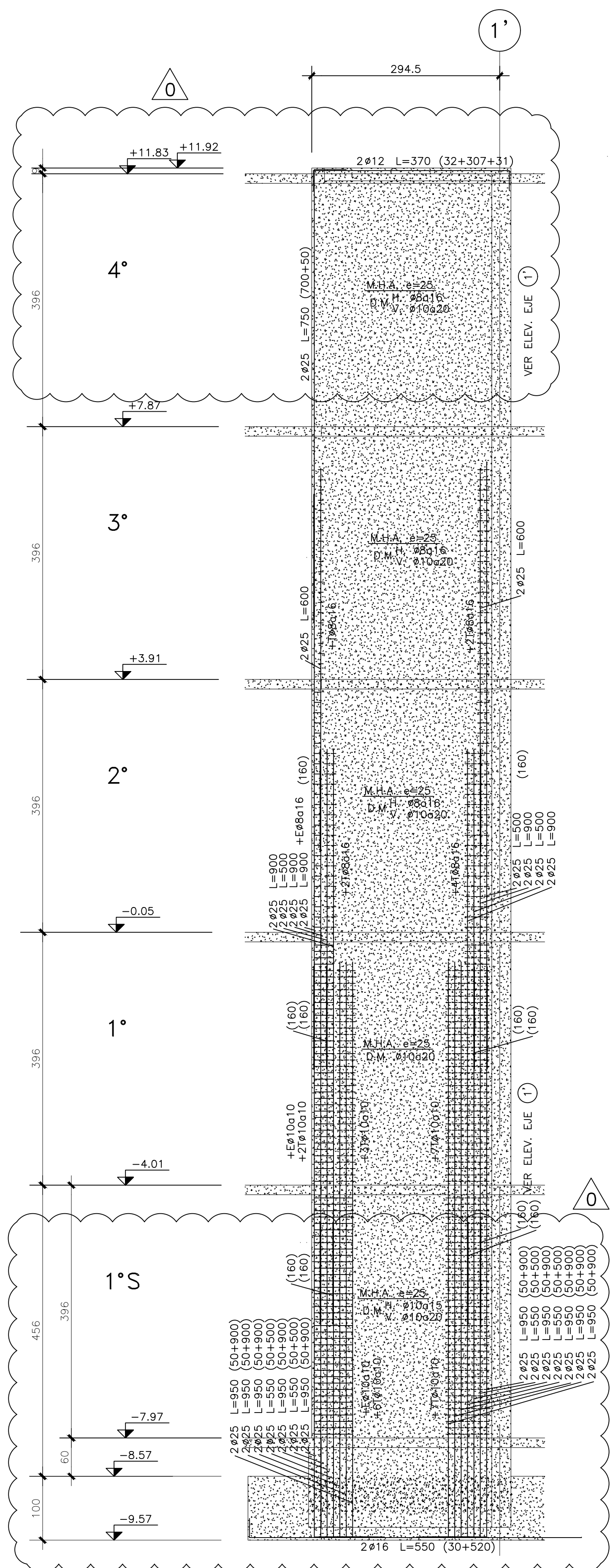
ELEVACION EJE C' ESCALA 1:50
