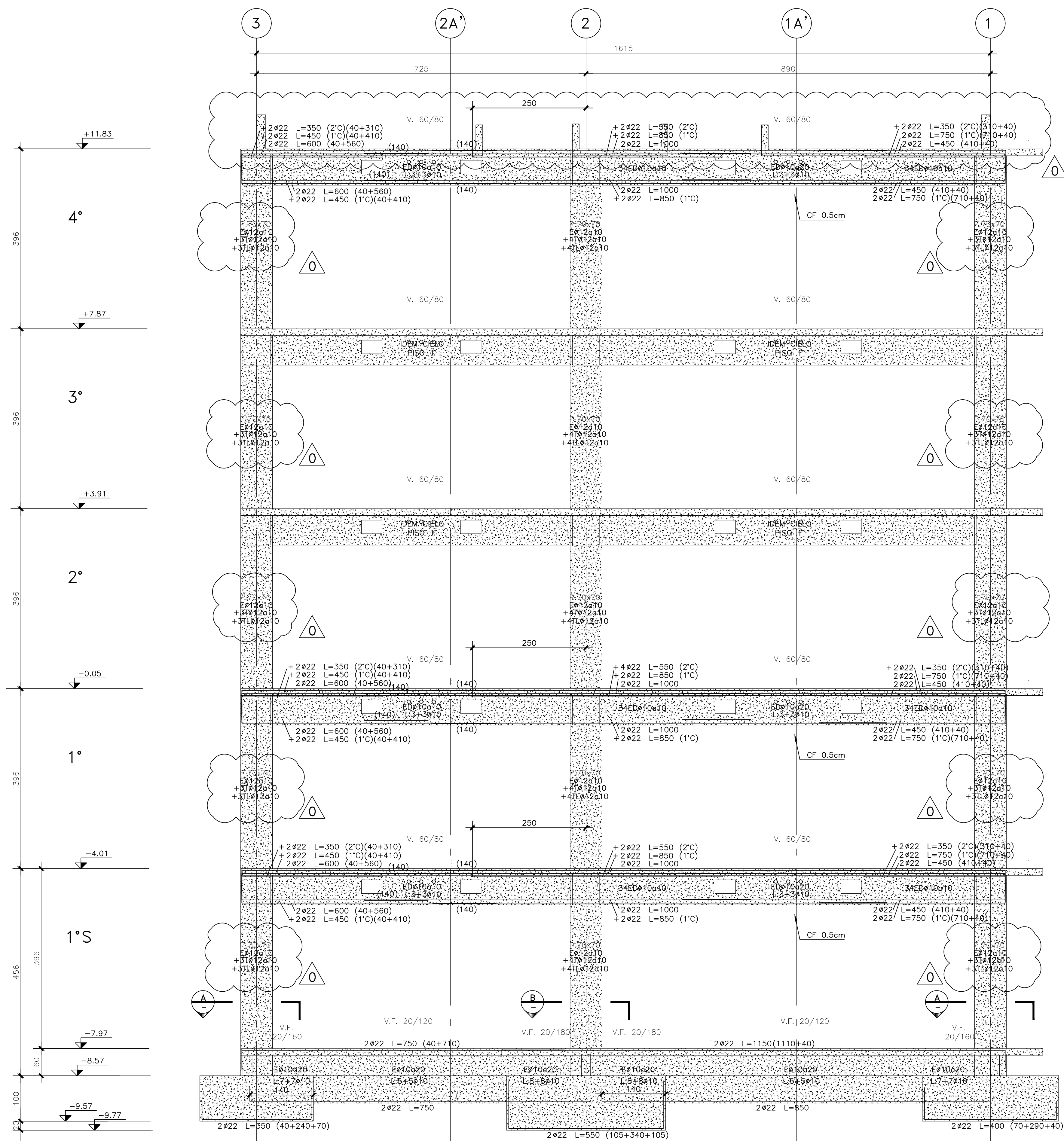
ELEVACION EJE B ESCALA 1:50
